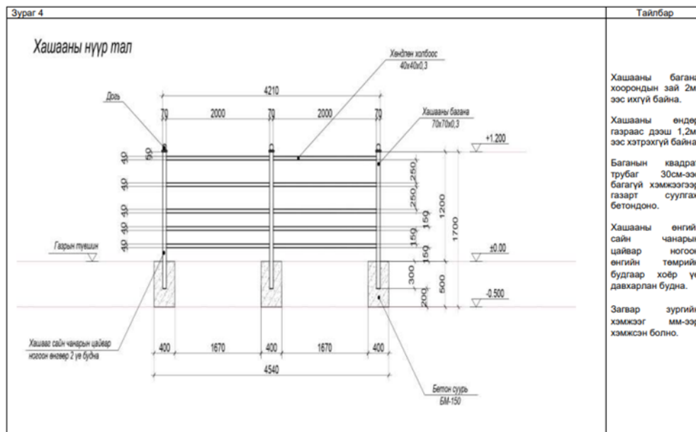
Зураг 32. Хамгаалалтын төмөр хашааны ажлын зураг
